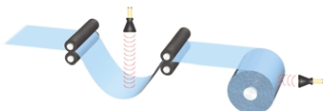
シートのループ・巻取制御
